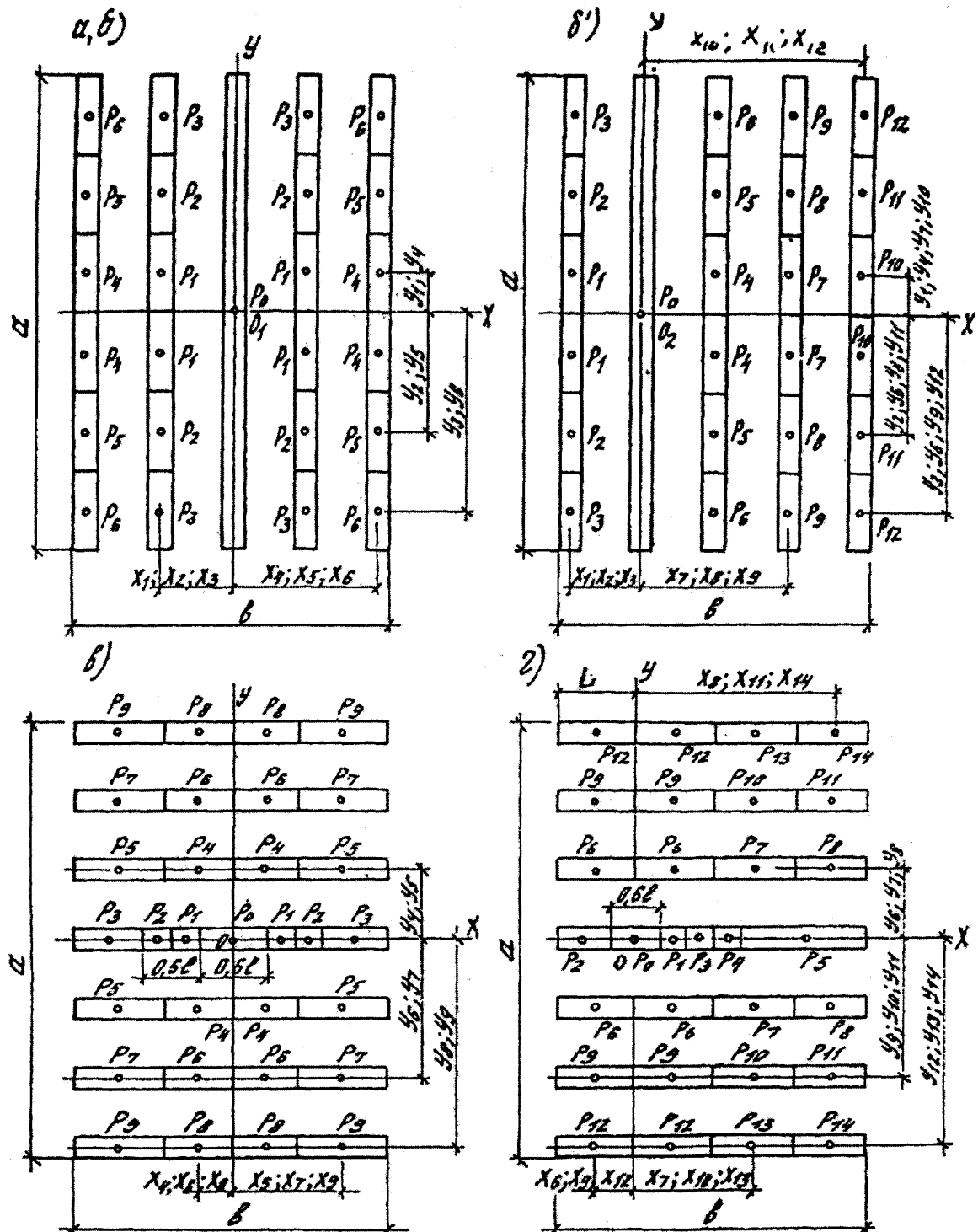
a, б – нагрузки, равномерно распределенные по длине параллельных следов (от прокладок под тяжелые предметы, от штабелей цилиндрических валов и др.) при b \leq 4,4l ; a > b ; б, б', з – то же, при b > 4,4l ; a > b
